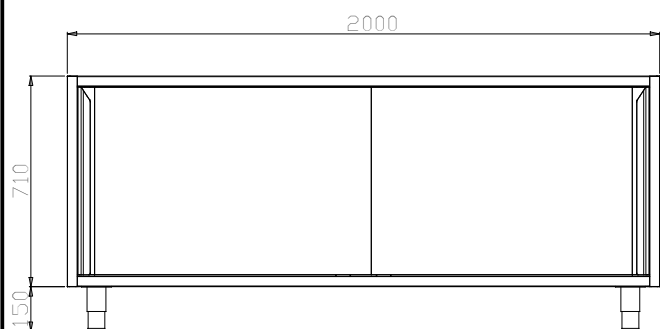
Alzado
